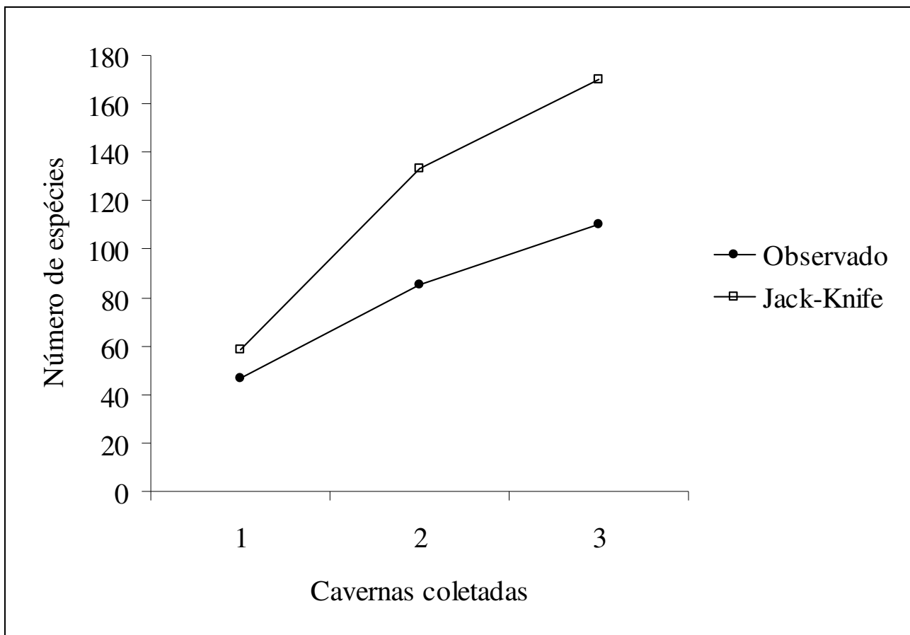
Figura 2. Curva acumulativa de espécies em função da quantidade de cavernas amostradas na PARNA de Ubajara (observado) e o número de espécies que se esperava encontrar (Jack-Knife).
