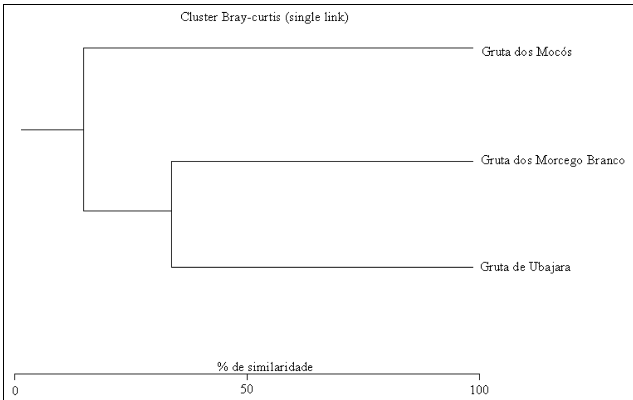
Figura 1. Similaridade qualitativa da fauna de invertebrados em três cavernas da PARNA de Ubajara, Ubajara, CE.
